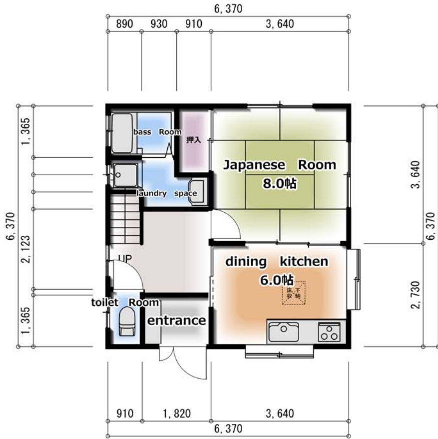
1階 縮尺 1/100
