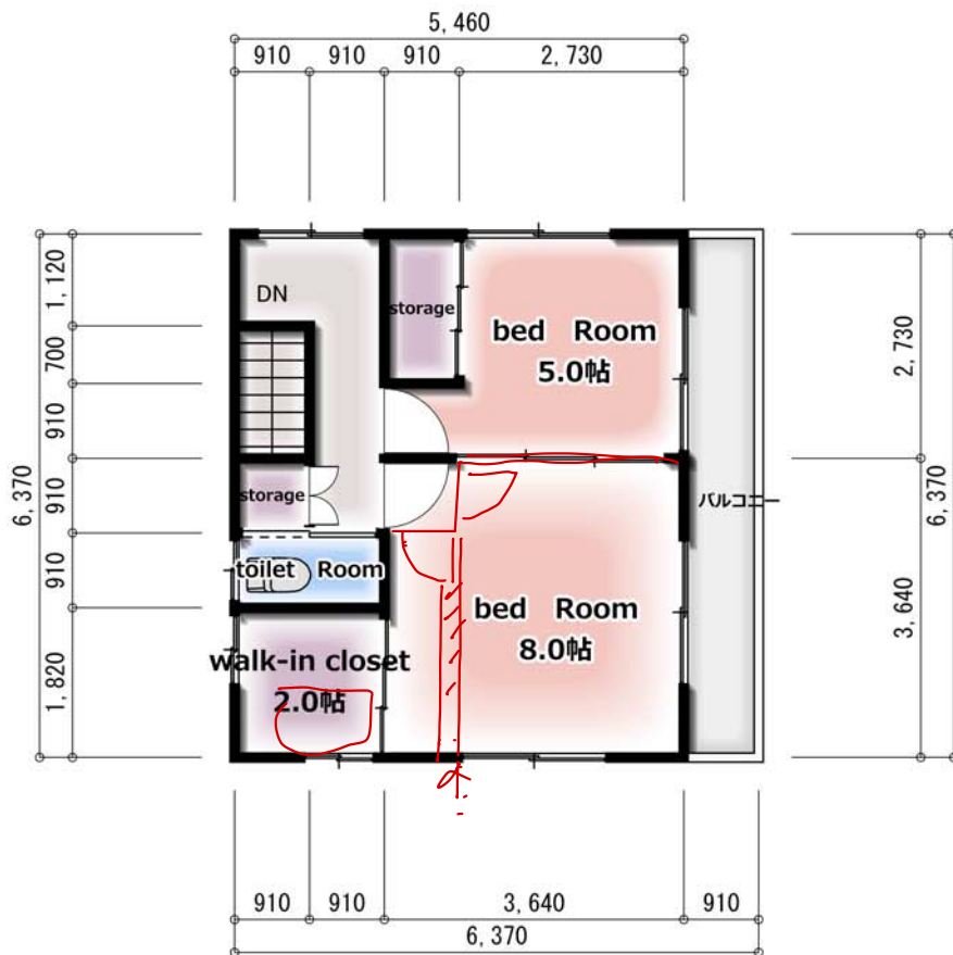
2階 縮尺 1/100
